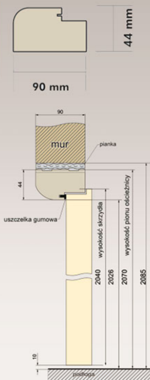
ościeżnica stała prestige
