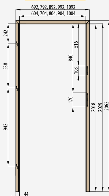
OŚCIEŻNICA STAŁA
