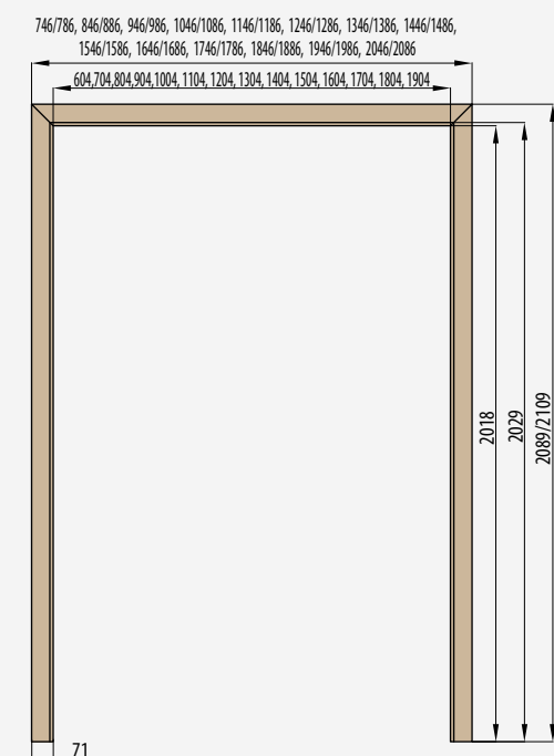
OŚCIEŻNICA REGULOWANA TYPU TUNEL opaska 6cm/opaska 8cm
