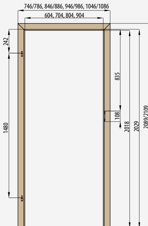
OŚCIEŻNICA REGULOWANA DO DRZWI SZKŁANYCH opaska 6 cm/opaska 8 cm
