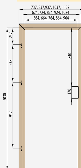
OŚCIEŻNICA NAKŁADKOWA
