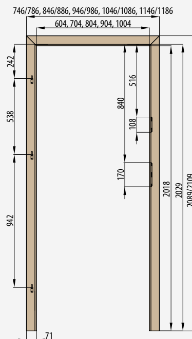
OŚCIEŻNICA REGULOWANA opaska 6cm/opaska 8cm
