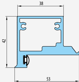
■ PRZEKRÓJ OŚCIEZNICY ALUMINIOWEJ
