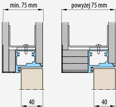
■ ZABUDOWA W MURZE
