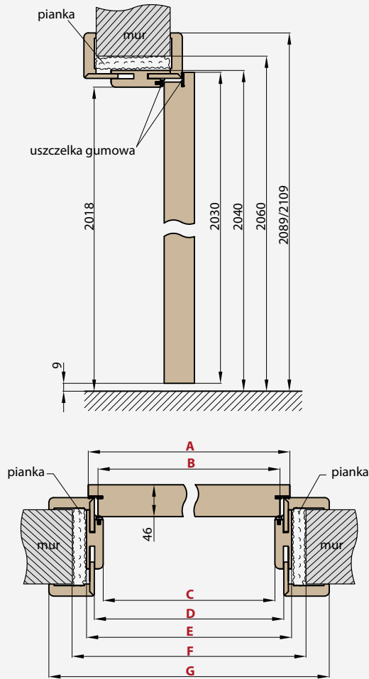
■ SCHEMAT OŚCIEŻNICY REGULOWANEJ HERSE SET
