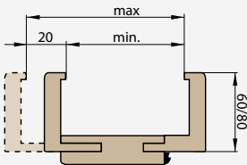
■ ZAKRĘS REGULACJI OŚCIEŻNICY REGULOWANEJ
