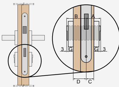
ZAMEK OSZCZĘDNOŚCIOWY
