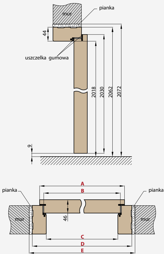
■ SCHEMAT OŚCIEŻNICY STAŁEJ HERSE SET
