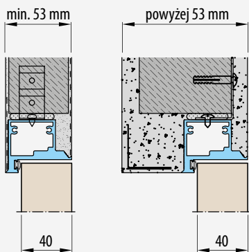
■ ZABUDOWA W MURZE
